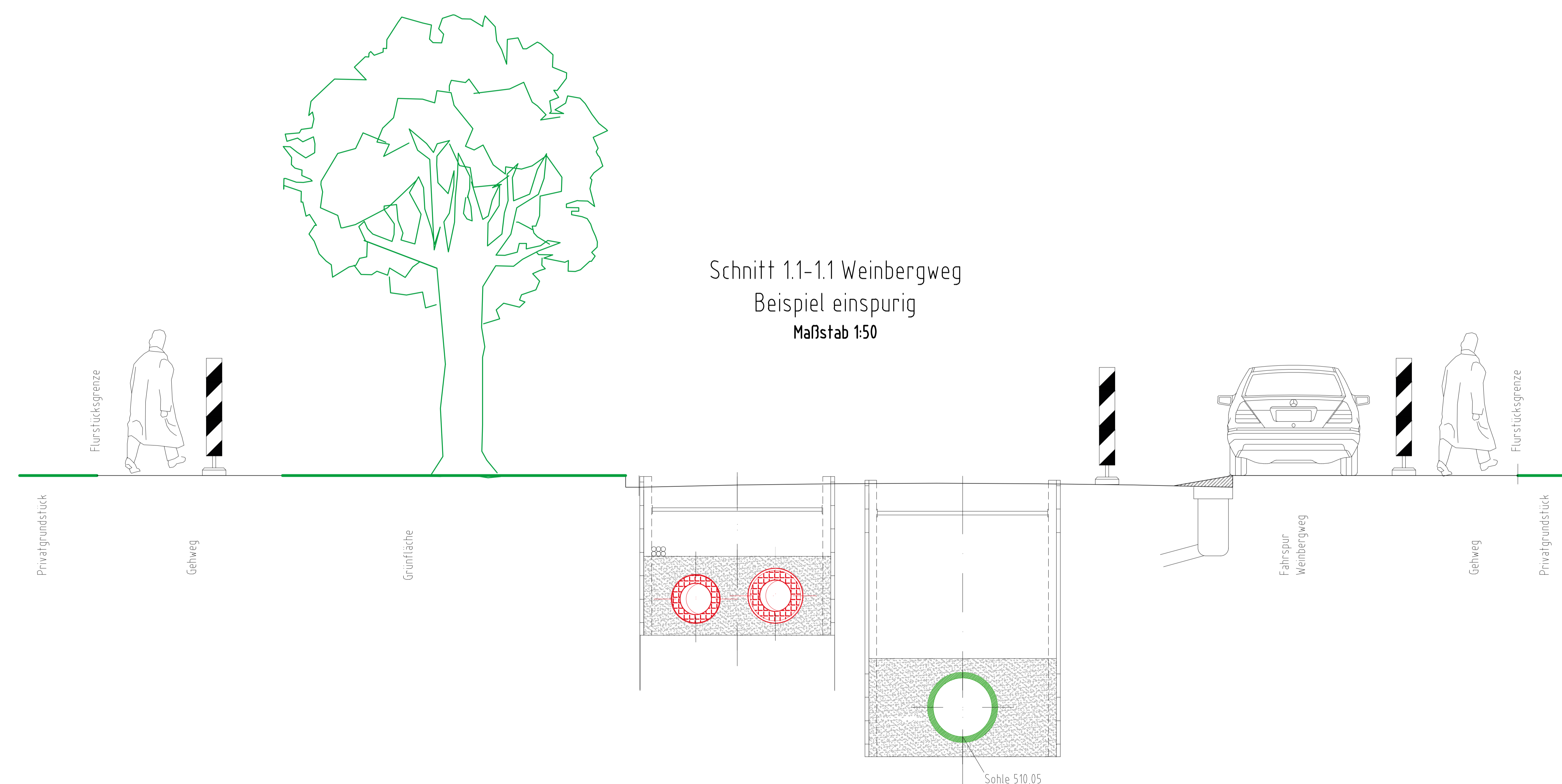
Trassenquerschnitt – Sanierung Abwasserkanal
